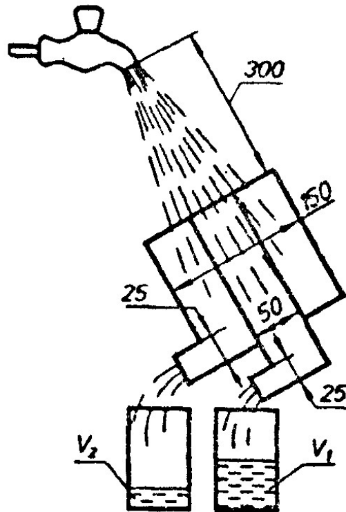
Рисунок 1 — Схема определения компактности струи
